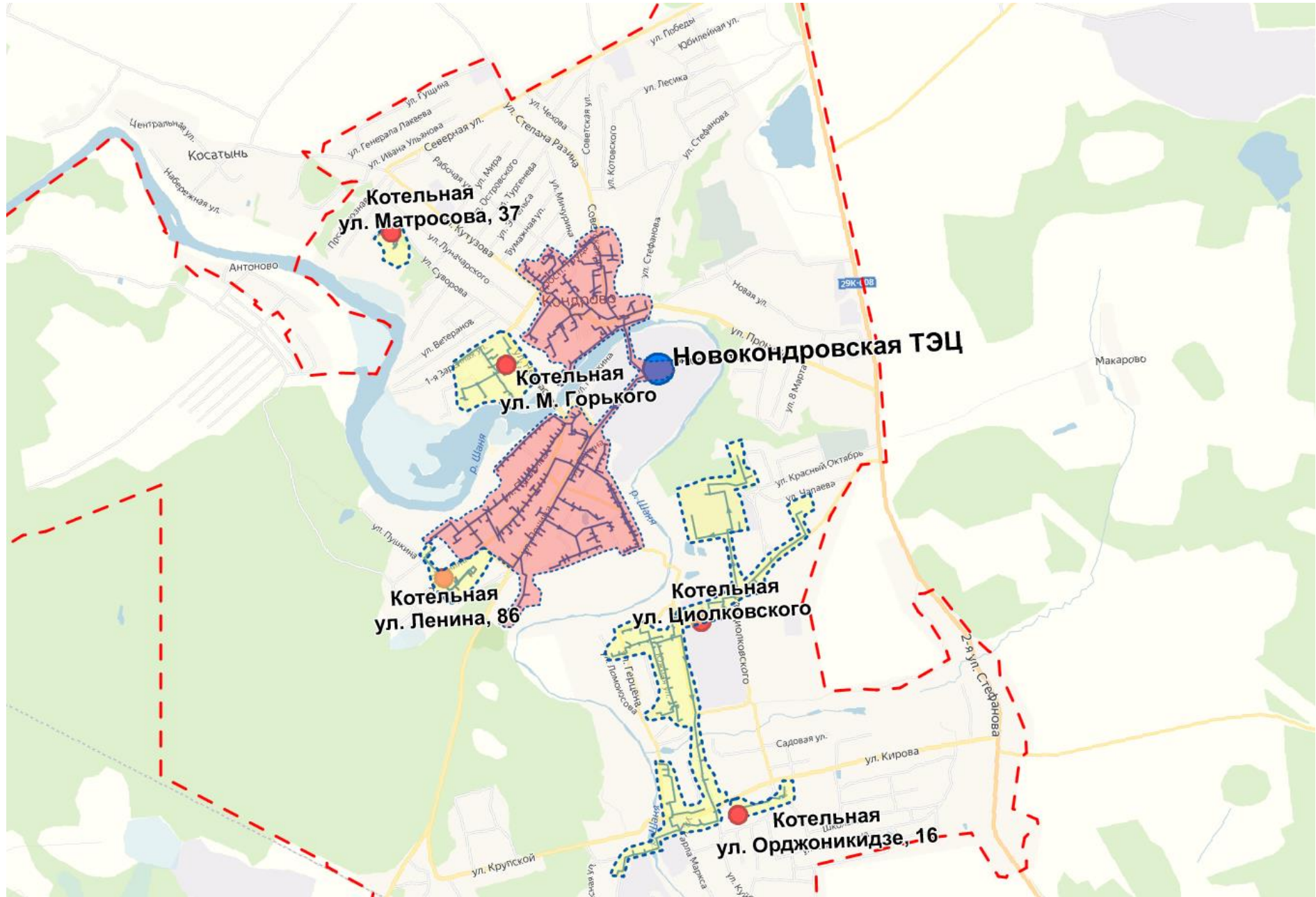
Рисунок 2.1.1-1 – Схема расположения теплоисточников на плане города и границы зон действия
