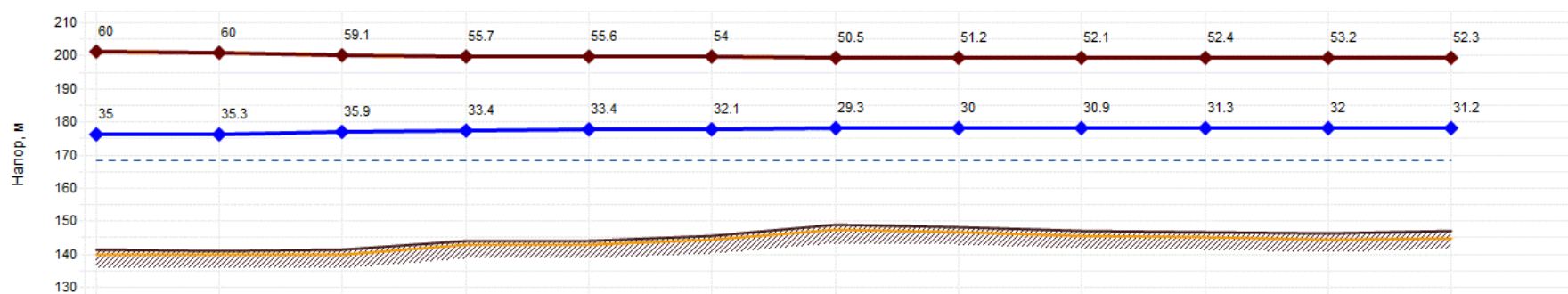
Рисунок 6.4-3 – Путь для построения пьезометрического графика участка от БМК-1 (Юг) до потребителя ул. Дзержинского, 3
