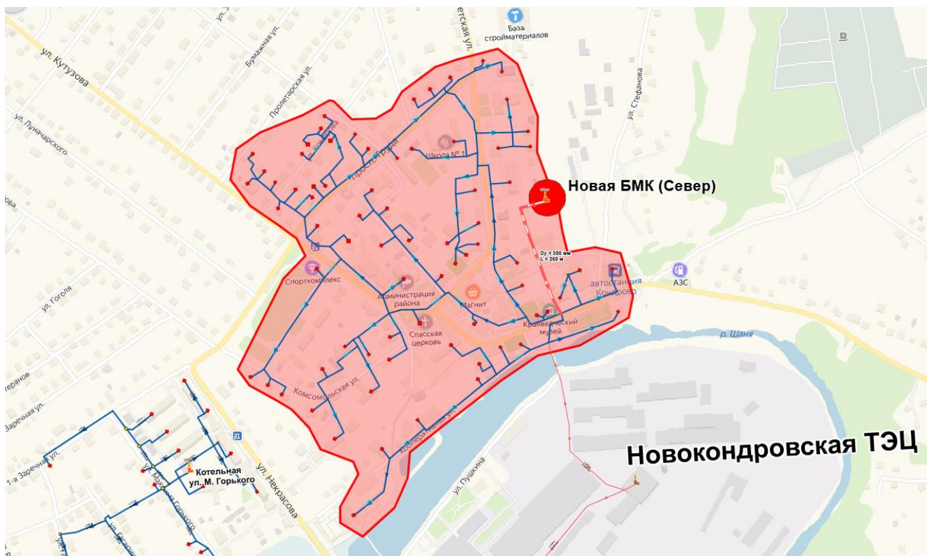
Рисунок 3.1-2 – Мероприятие по строительству БМК-2 (Север) вместо Новокондровской ТЭЦ
