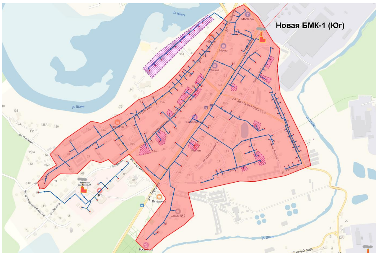
Рисунок 3.1-1 – Мероприятие по строительству БМК-1 (Юг) вместо Новокондровской ТЭЦ
