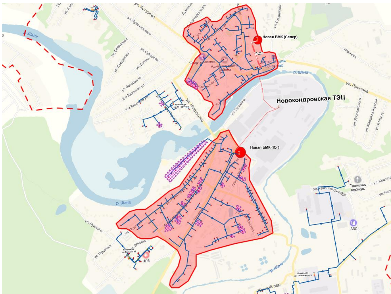
Рисунок 5.1.2-1 - Переключаемые зоны
